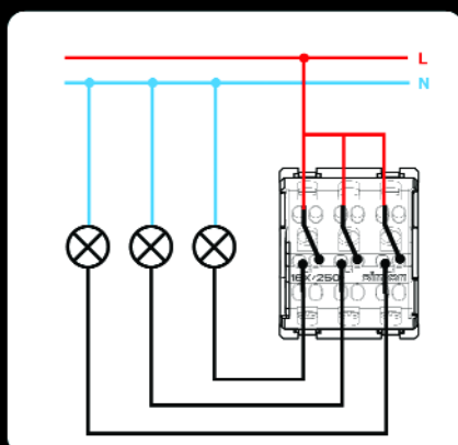
Выключатель трехклавишный
