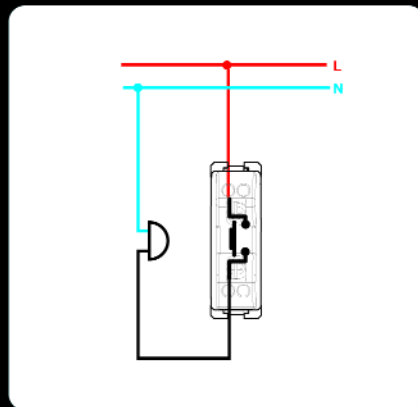
Клавишная кнопка
