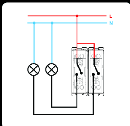
Двойной выключатель
